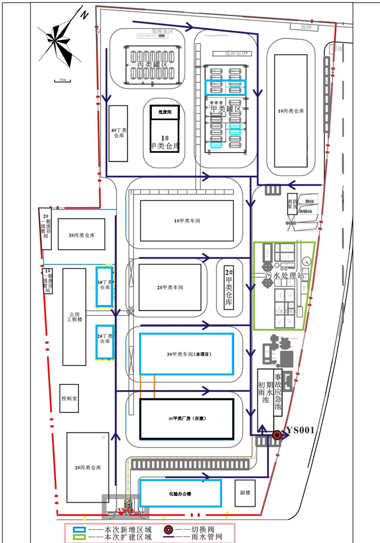
附图 7 项目厂区雨水管网图
