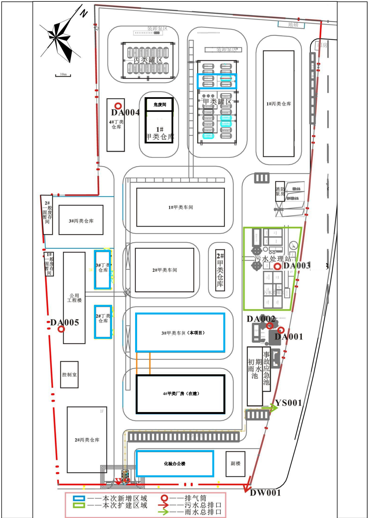
附图3 项目厂区平面布置图
