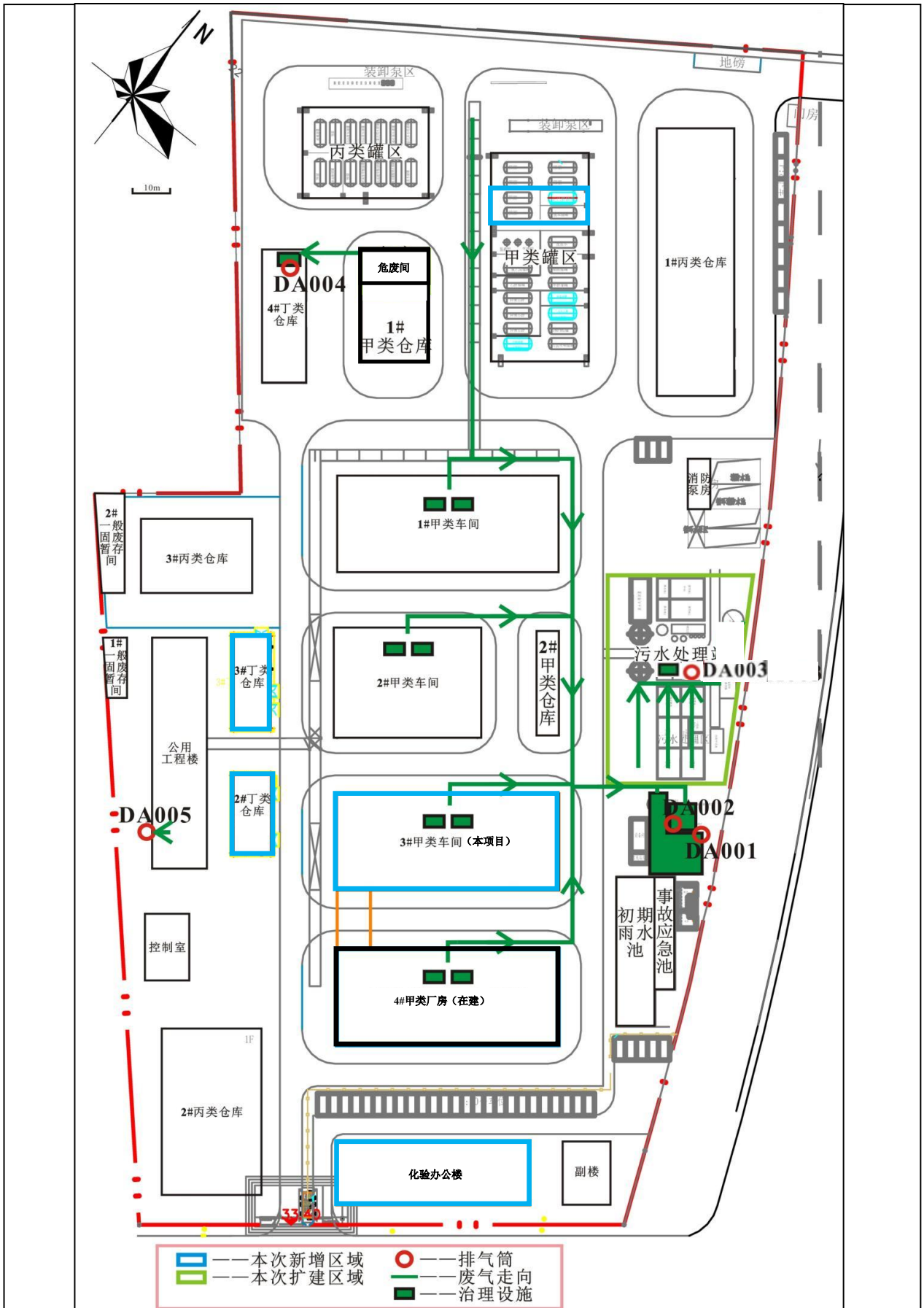
附图5 项目厂区废气走向图
