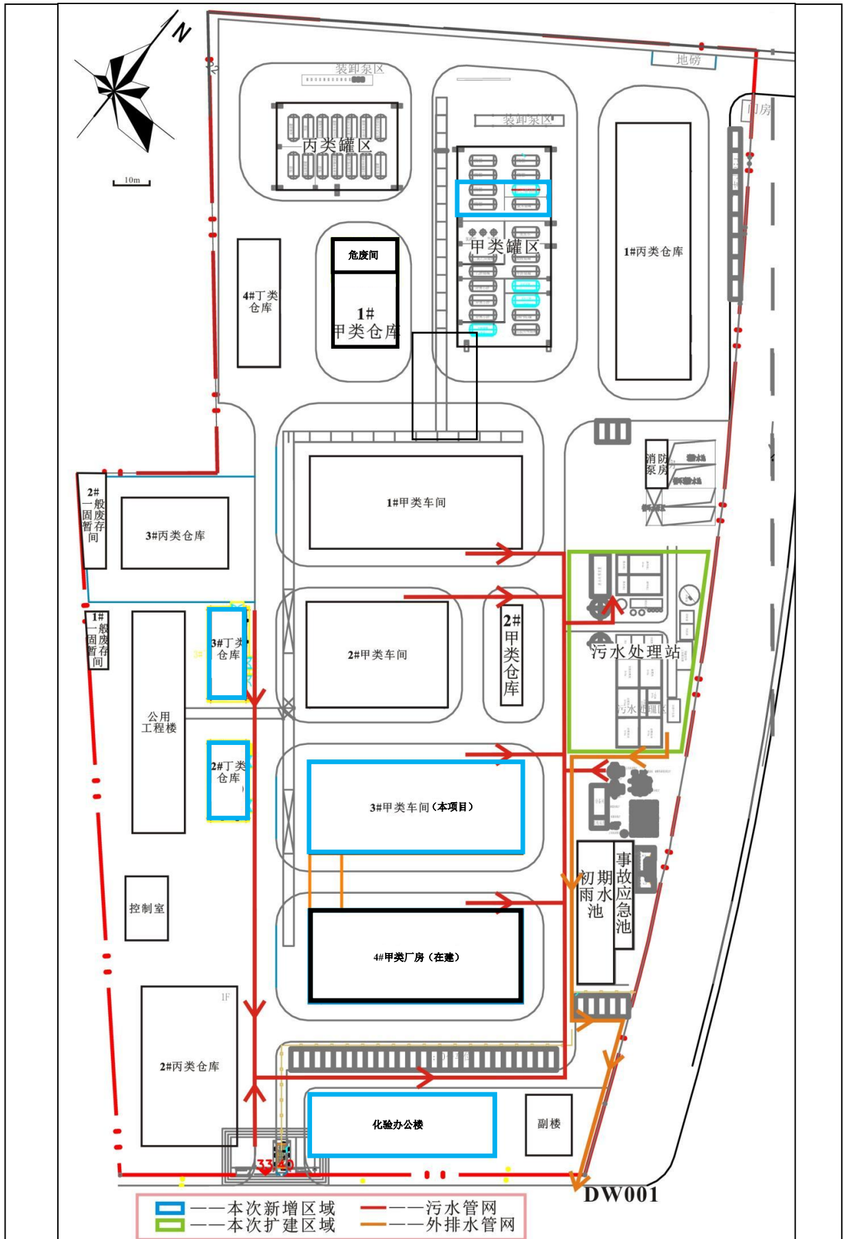
附图6 项目厂区污水管网图
