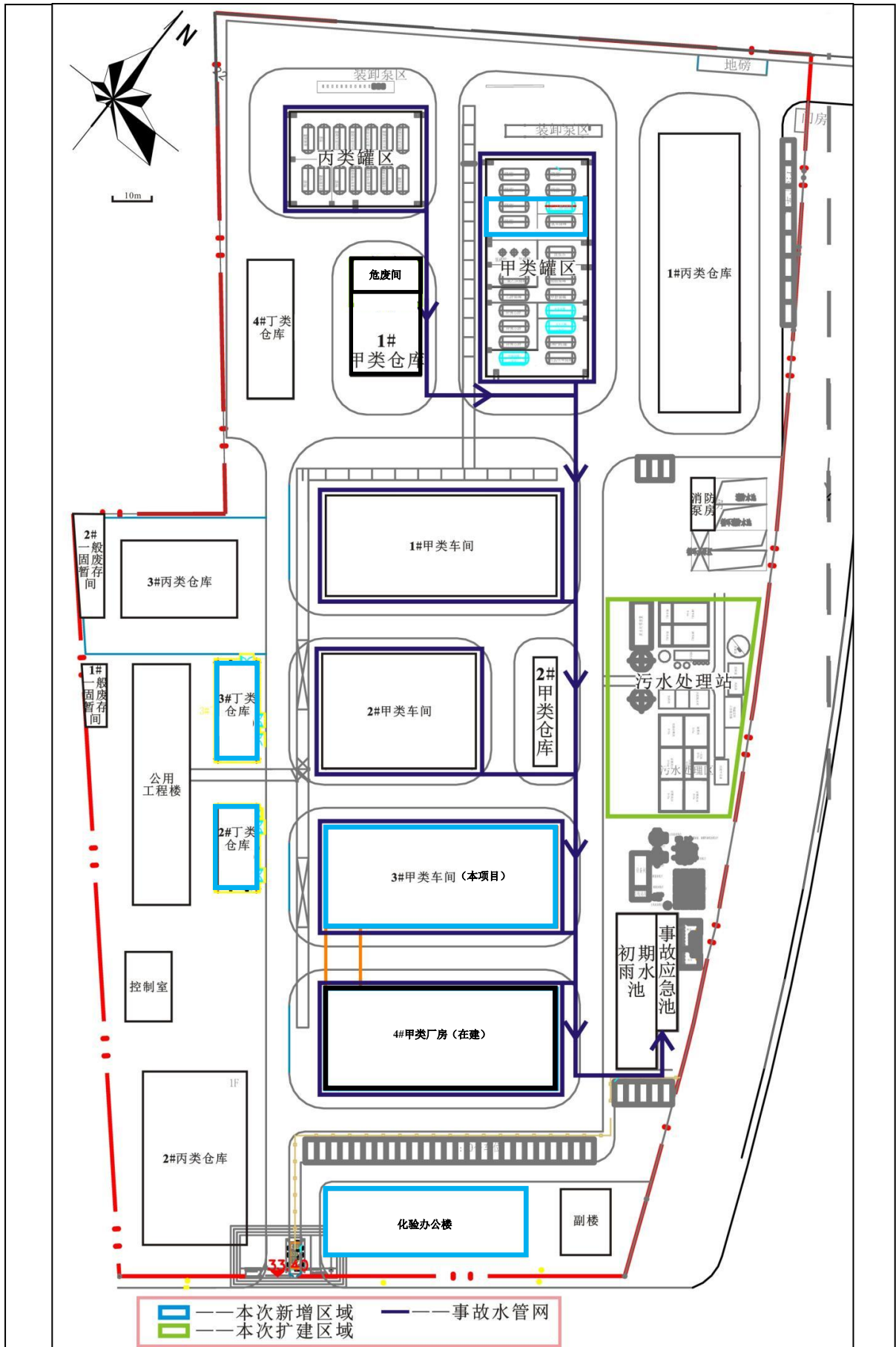
附图 8 项目厂区事故管道布置图
