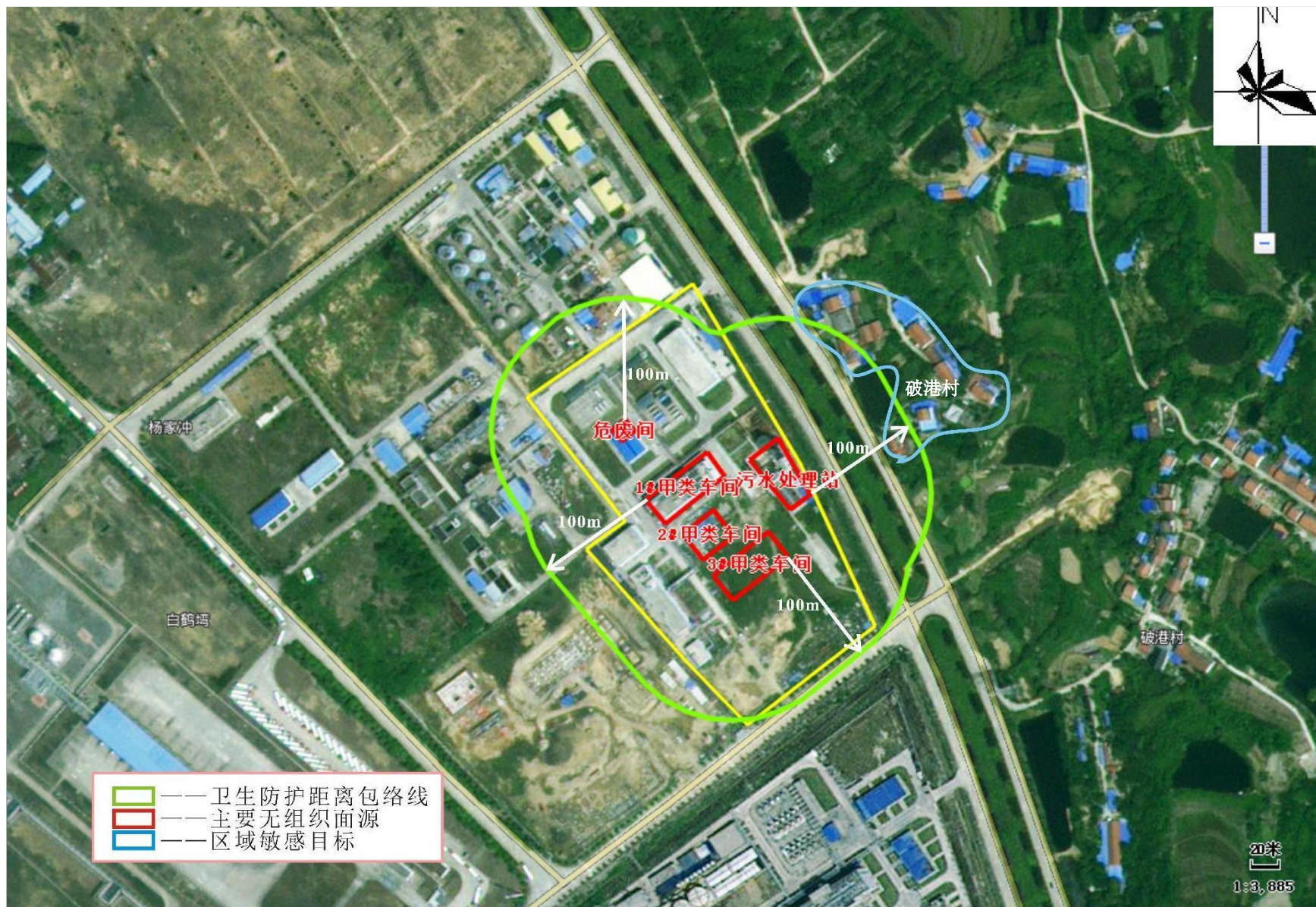
附图 10 卫生防护距离包络线图
